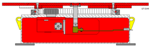
Posicionador Horizontal 20Tn
