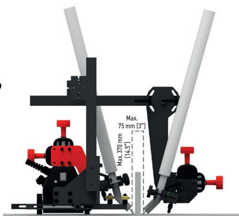
Ensamble doble antorcha PDT-0466-40-00-00-0
