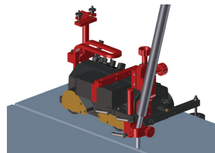
Soldadura a tope con oscilador
