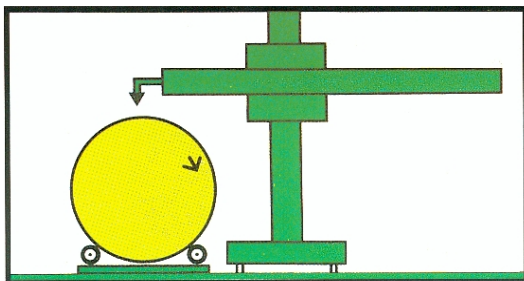
(1) Soldadura externa circunferencial. Puede realizarse con columna fija.
