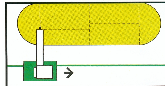
(2) Soldadura externa longitudinal. La columna recorre toda la longitud del depósito.
