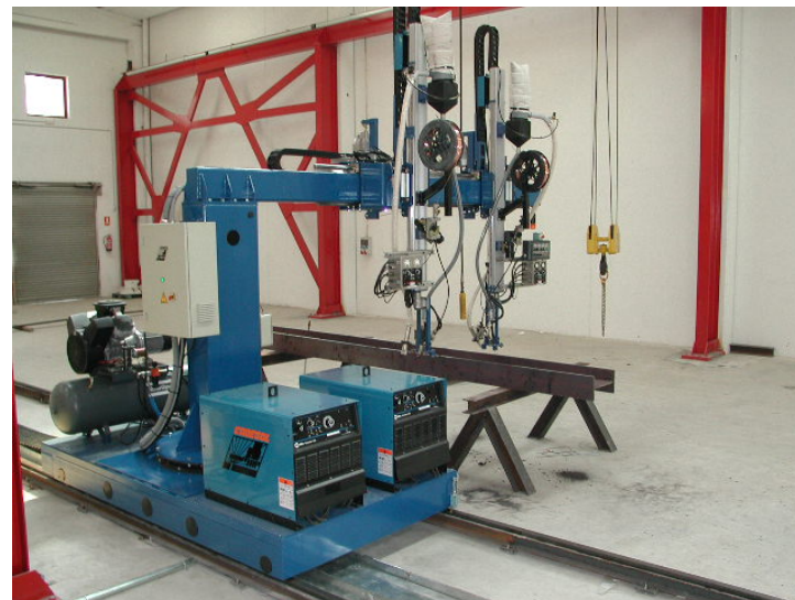
PILARES doble UPN
