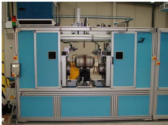
Soldadura Mig Pulsado – 3 arcos de soldadura simultáneos (cierre botella, asa y base de la botella)
